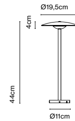
Ginger B Ground fixation plate · Placa de fijación al suelo
